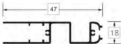
Prowadnica Prosta:
