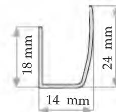
Prowadnica przestrzenna
