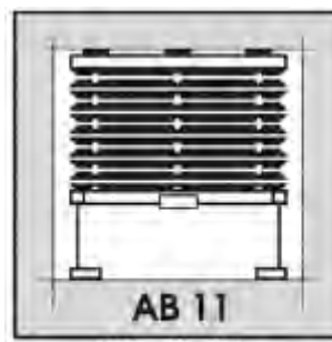
AB 11 MAX. width 150cm MAX. high 250cm
