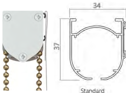
Szyna do rolety rzymskiej:
