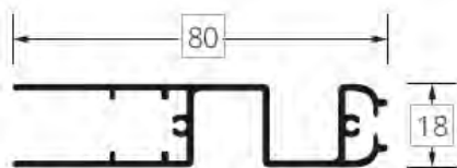
Profil Moskitiery :
