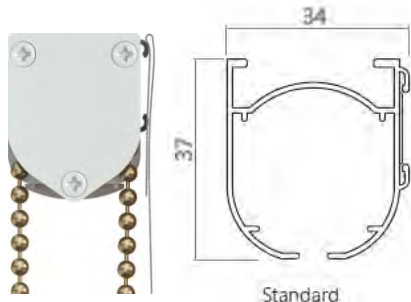
Szyna do rolety rzymskiej:
