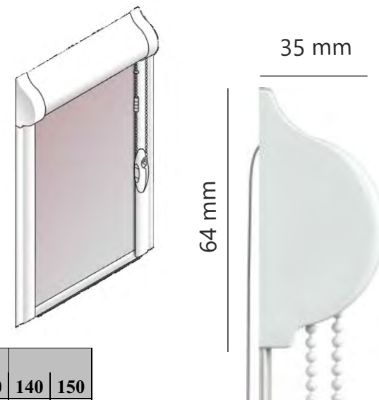
Prowadnica płaska
