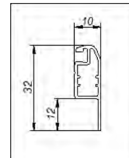
Nowy Profil:
