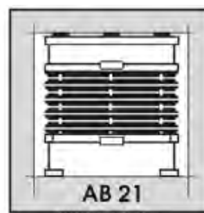
AB 21 MAX. width 150cm MAX. high 250cm
