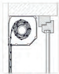
Typ „A” Roleta zamontowana we wnęce okna (prawoskrętna).
