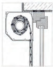
Typ „B” Roleta zamontowana we wnęce okna (lewoskrętna).
