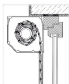
Typ „B” Roleta zamontowana we wnęce otw. (lewyoskrętna).
