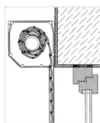
Typ „C” Roleta zamontowana na ścianie budynku (lewyoskrętna).
