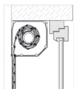
Typ „A” Roleta zamontowana we wnęce otw. (prawyoskrętna).
