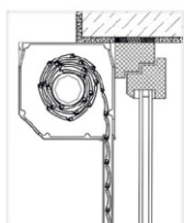
Typ „B” Roleta zamontowana we wnęcie okna (levoskrętna).
