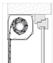
Typ „A” Roleta zamontowana we wnęcie okna (prawoskrętna).
